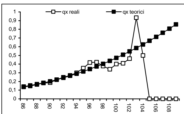
Graf. A.3.1 Curva teorica di interpolazione delle probabilità di morte (MASCHI) – 86 anni ed oltre
