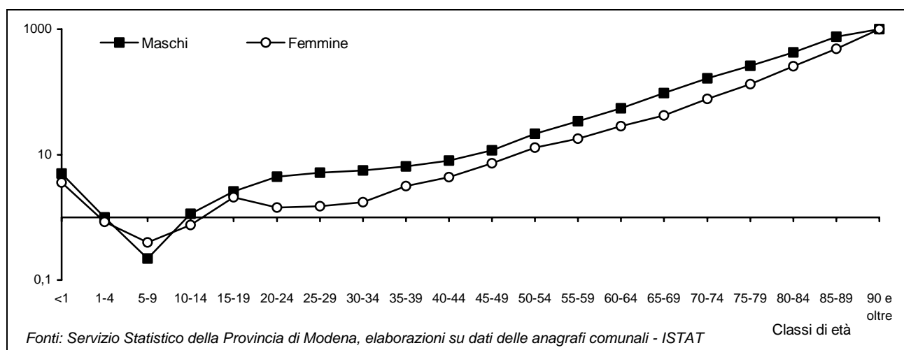
Graf.2.I Probabilità di morte q_x \cdot 1.000 per classi quinquennali di età - tavola di mortalità abbreviata della provincia di Modena - Periodo 1997-2001 (scala logaritmica) - Valori %
