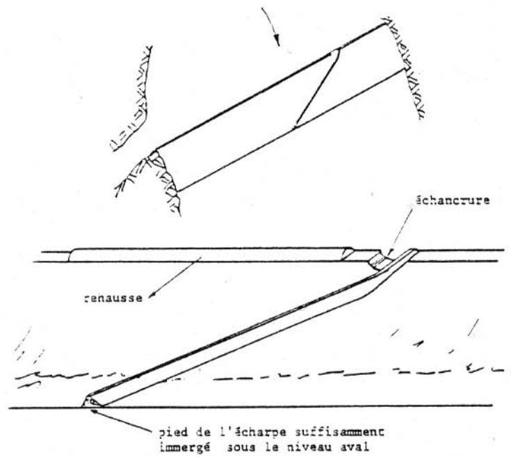
Figure 7 : Passe en écharpe
