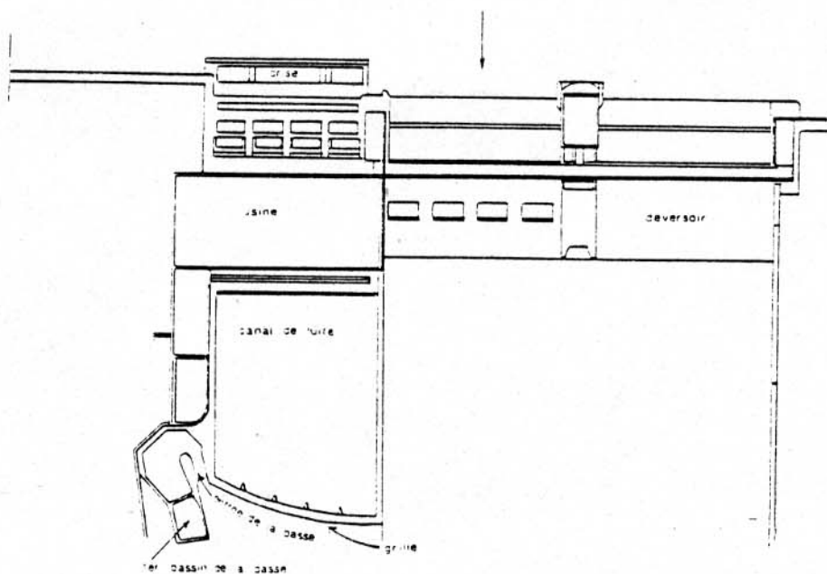
Figure 2 : Implantation d'une passe dans un aménagement hydroélectrique. Exemple de Pîtres en Écosse.
