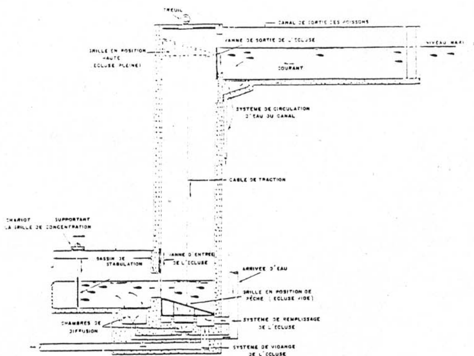
Figure 12: Schéma de principe d'une écluse à poissons munie d'un système obligeant les migrateurs à passer à l'amont (d'après RIZZO)
