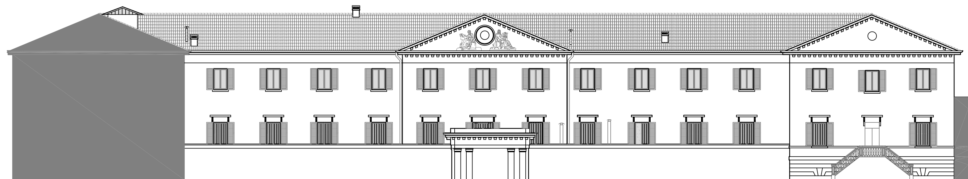
PROSPETTO SUD
