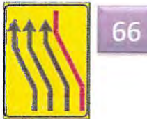
Figura II 412/f Art. 43 SEGNALE DI RIENTRO IN CARREGGIATA
